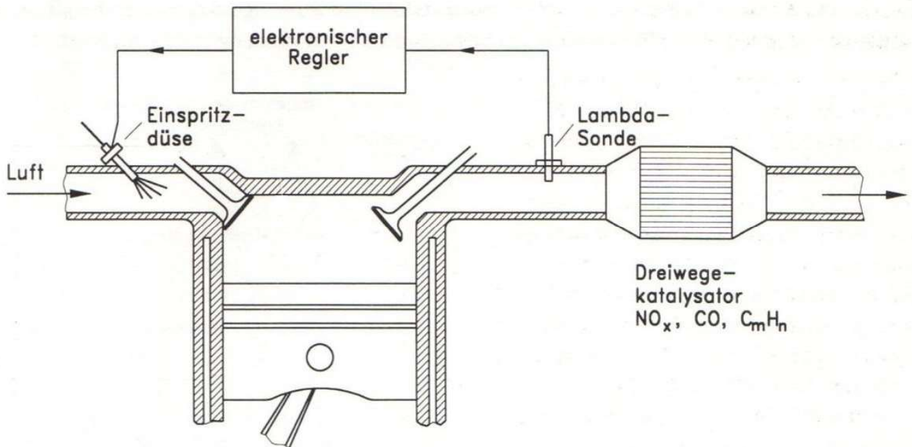
Abb. 5.8: Das Prinzip der Lambda-Regelung
