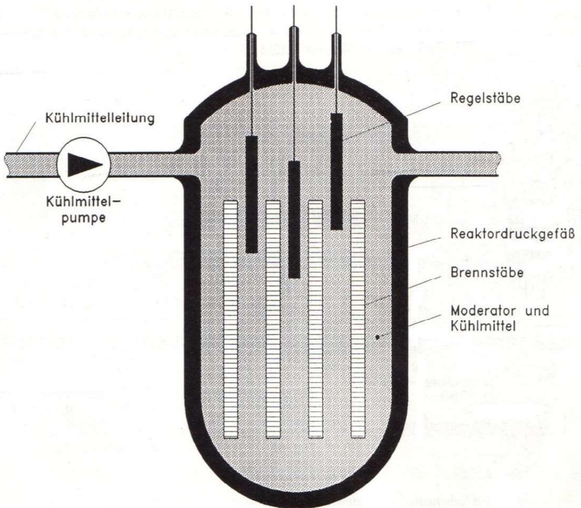
Abb. 4.42: Aufbau eines Leichtwasserreaktors (Prinzip)
