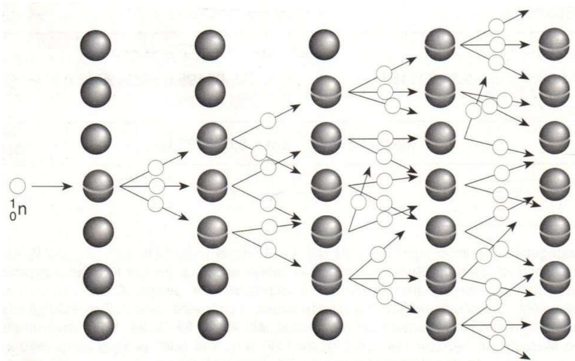
Abb. 4.40: Schematische Darstellung einer Kettenreaktion
