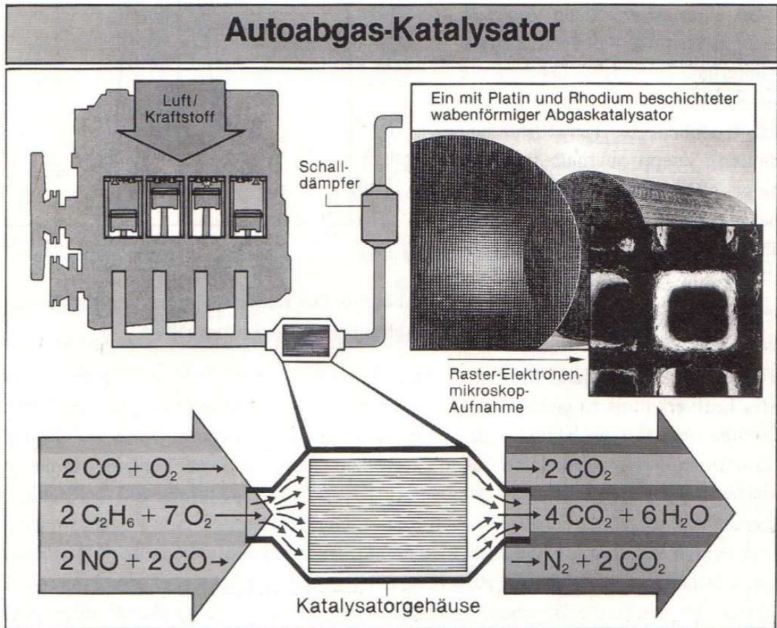
Abb. 5.6: Aufbau und Funktionsweise eines Dreiwegekatalysators
