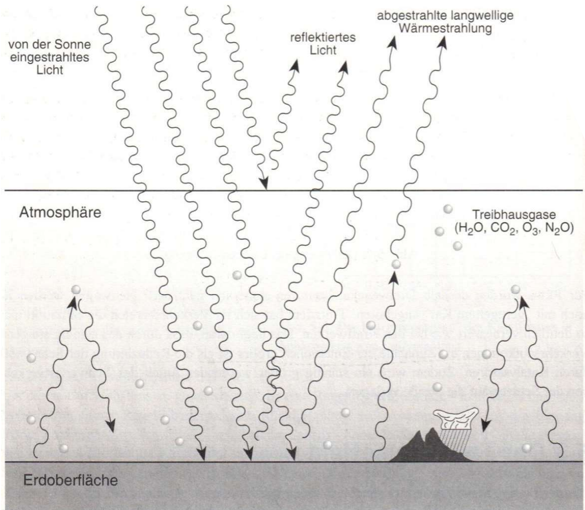
Abb. 5.9: Schematische Darstellung des Treibhauseffektes
